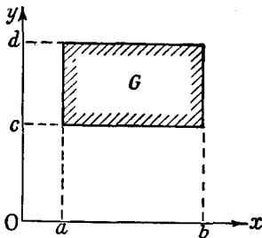
Fig. 3.—A rectangular region
