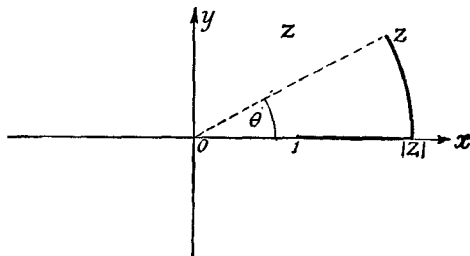
Fig. 4.— \log z = \log |z| + i\theta
