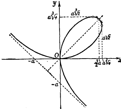
Fig. 3.—Folium of Descartes
