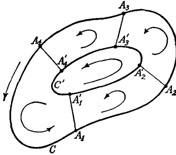
Fig. 2.— \sum_{i=1}^n \int_{o_i} = \int_{o'} - \int_{o''}
