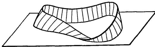
Fig. 9.—The Möbius band
