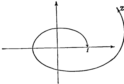
Fig. 5.— \log z = \log |z| + i\theta + 2\pi i
