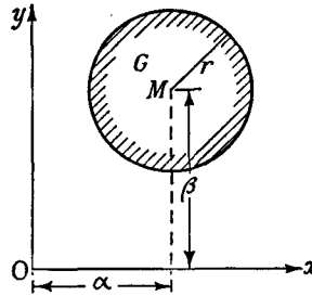
Fig. 4.—A circular region
